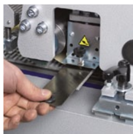
Slipdyna för finslipning inkluderar quick change system
