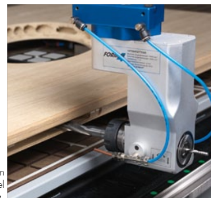
C-axeln står till förfogande som en fjärde interpolerande (360°) axel med tryckluftsanslutning.
